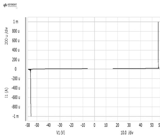
Figure4: I-V Curve
